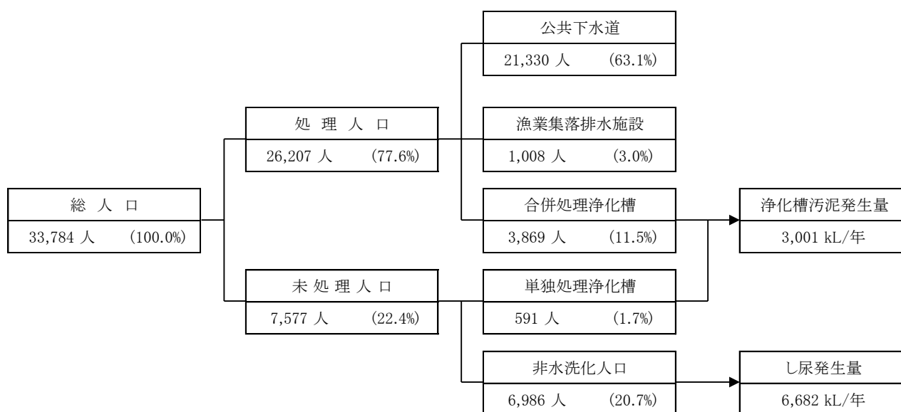
図 2-3 生活排水処理の処理状況フロー（平成 30 年度）
