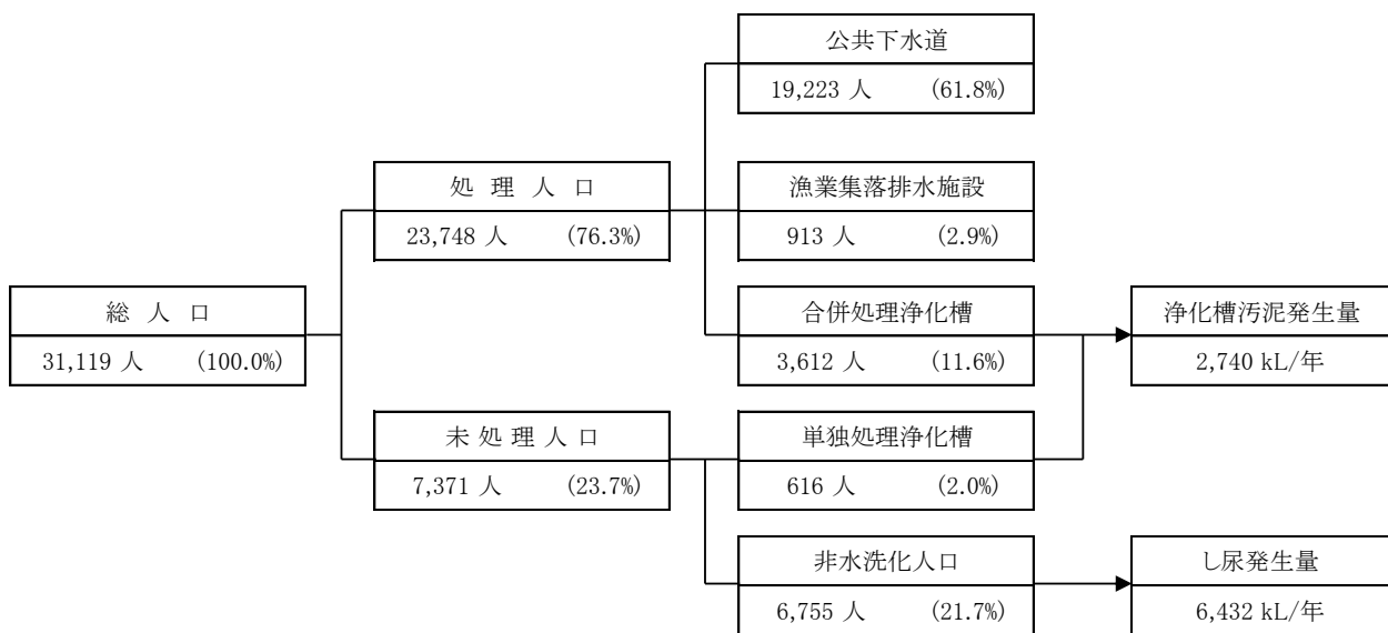
図 2-7 生活排水処理の処理状況フロー（令和 7 年度）
